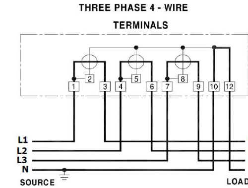
รูปที่ 2.3 การต่อสายไฟเมนและสายไฟโหลด
